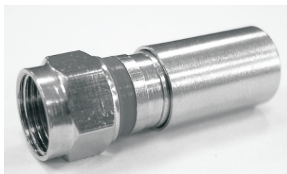
CNF50010 Conector "F" compressão RG-59
