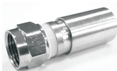
CNF60012 Conector "F" compressão RG-6
